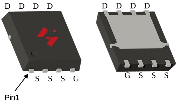
PDFN8L(5X6)
